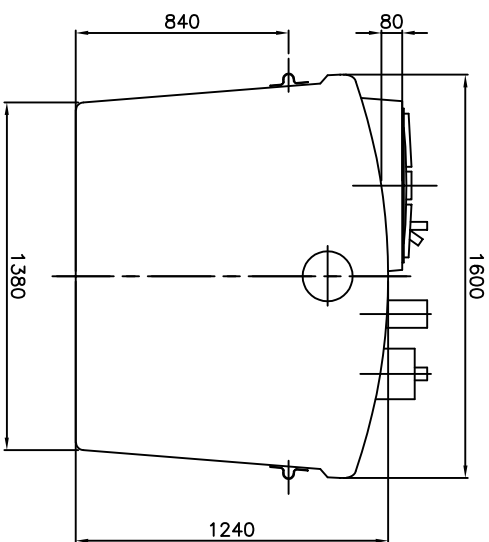
DETALLE OREJA DE ELEVACION TIPO DE OREJAS: OMEGA
