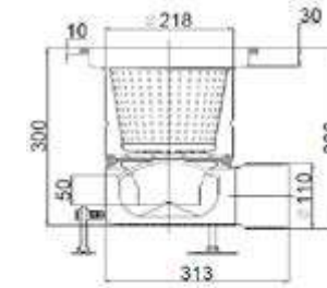
EG con Cestillo Extendido Fijo com Cesto Estendido Fixo 300x300mm DN110 Salida Horizontal Saída Horizontal
