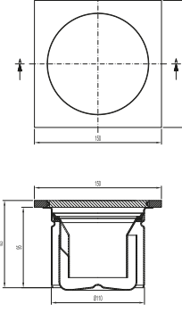
Sumidero EG150 Estanco Sumidouro EG150 Estanque
