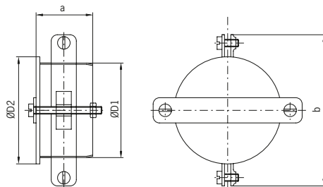
Tapón con abrazadera Tampão com braçadeira
