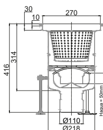
EG con Cestillo Extendido Fijo com Cesto Estendido Fixo 300x300mm DN110 Salida Vertical Saída Vertical
