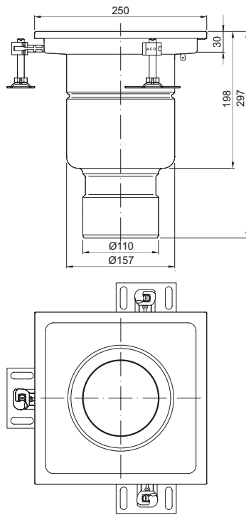
EG Fijo Fijo 250x250mm DN110 Salida Vertical Saída Vertical
