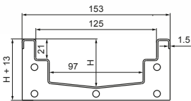
Canal Modular CM125 Canal Modular 125
