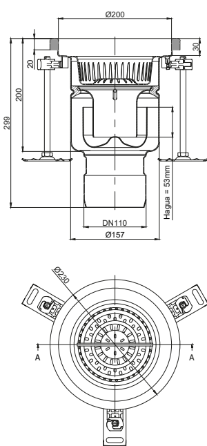
EG Fijo Fixo ø230mm DN110 Salida Vertical Saída Vertical
