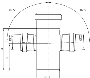
Derivación doble 87,5° con reducción Derivação duplo 87,5° com redução
