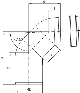
Codo de extensión de 87,5° Curva de extensão de 87,5°
