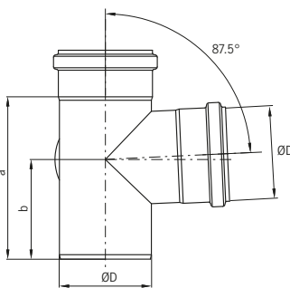
Esquina derivación doble 87,5° Canto derivação duplo 87,5°
