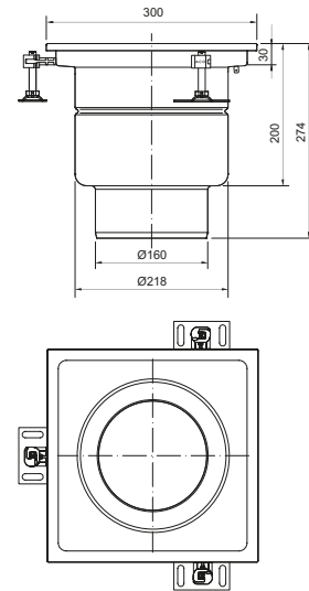
EG Fijo Fijo 300x300mm DN160 Salida Vertical Saída Vertical
