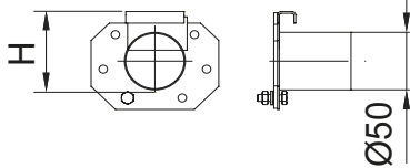
Tapa Final con Salida DN50 Tampa de fim com Saída DN50
