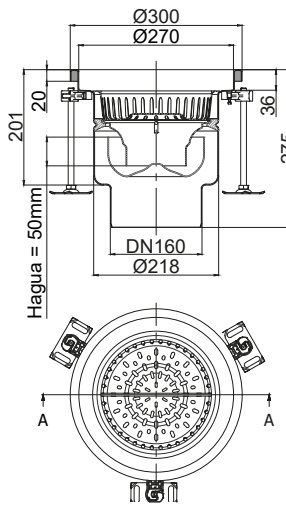
EG Fijo Fijo ø300mm DN160 Salida Vertical Saída Vertical
