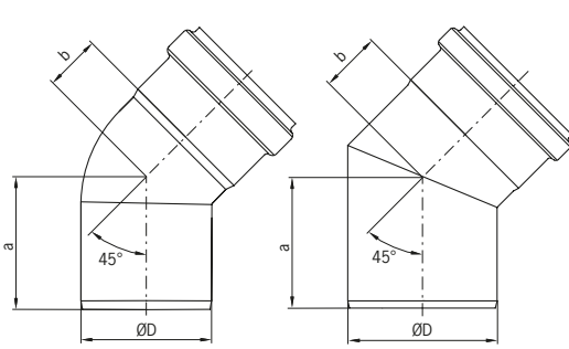
Codo de 45° Curva de 45°
