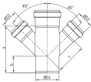
Derivación doble 45° con reducción Derivação suplo 45° com redução
