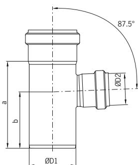
Derivación simple 87,5° con reducción Derivação simple 87,5° com redução
