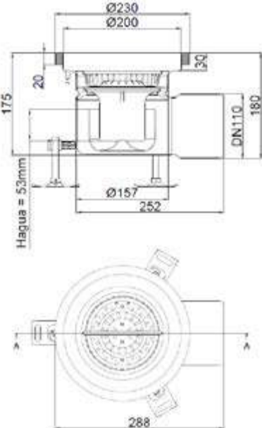
EG Fijo Fixo ø230mm DN110 Salida Horizontal Saída Horizontal
