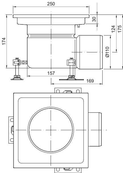
EG Fijo Fijo 250x250mm DN110 Salida Horizontal Saída Horizontal
