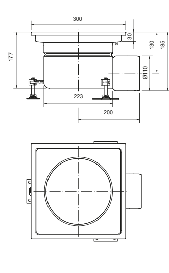
EG Fijo Fijo 300x300mm DN110 Salida Horizontal Saída Horizontal
