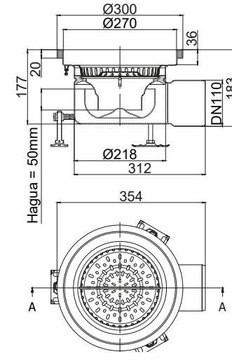
EG Fijo Fijo ø300mm DN110 Salida Horizontal Saída Horizontal
