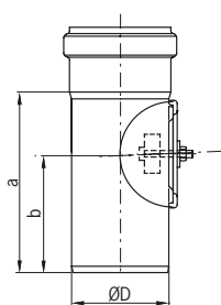
Unidad de acceso Unidade de acesso
