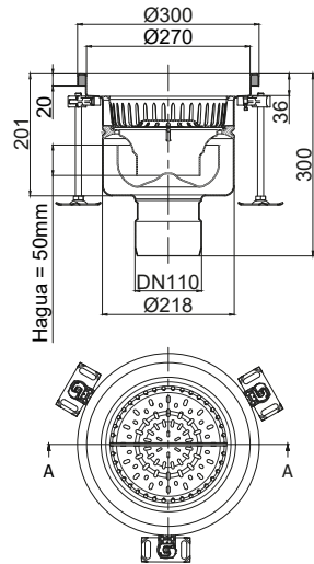
EG Fijo Fijo ø300mm DN110 Salida Vertical Saída Vertical
