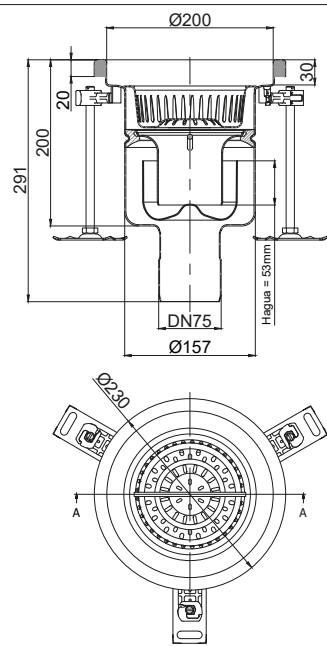
EG Fijo Fixo ø230mm DN75 Salida Vertical Saída Vertical
