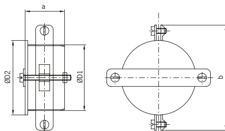
Tapón con abrazadera Tampão com braçadeira
