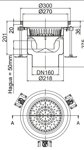
EG Fijo Fixo ø300mm DN160 Salida Vertical Saída Vertical
