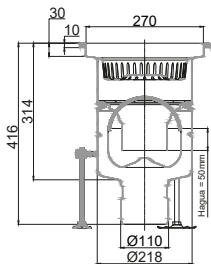
EG con Sifón Extendido Fijo com Sifão Estendido Fijo 300x300mm DN110 Salida Vertical Saída Vertical
