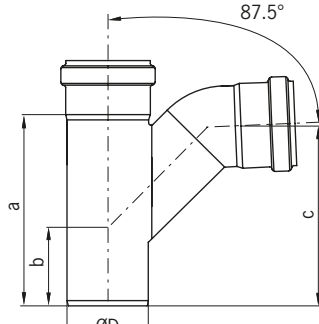
Derivación simple con codo 45° Derivação simple com curva 45°
