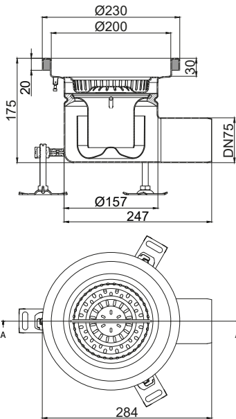
EG Fijo Fixo ø230mm DN75 Salida Horizontal Saída Horizontal
