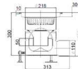
EG con Sifón Extendido Fijo com Sifão Estendido Fijo 300x300mm DN110 Salida Horizontal Saída Horizontal
