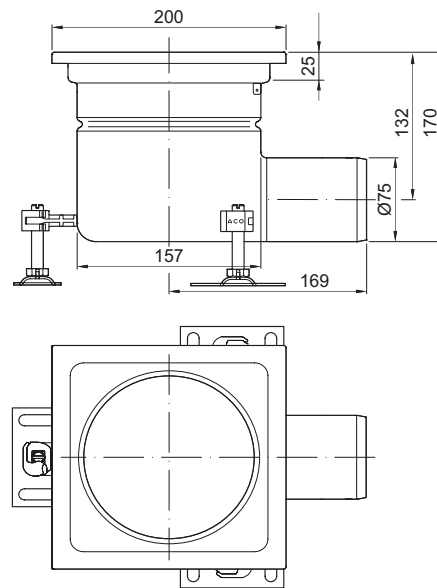
EG Fijo Fijo 200x200mm DN75 Salida Horizontal Saída Horizontal
