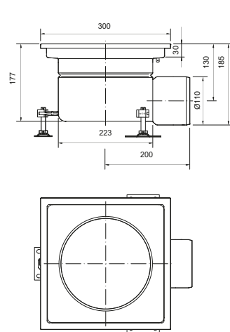
EG Fijo Fijo 300x300mm DN110 Salida Horizontal Saída Horizontal
