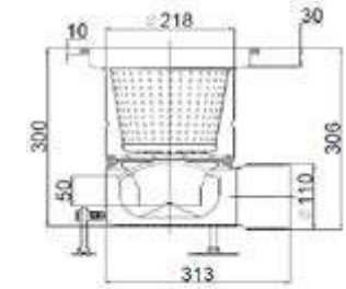
EG con Cestillo Extendido Fijo com Cesto Estendido Fijo 300x300mm DN110 Salida Horizontal Saída Horizontal
